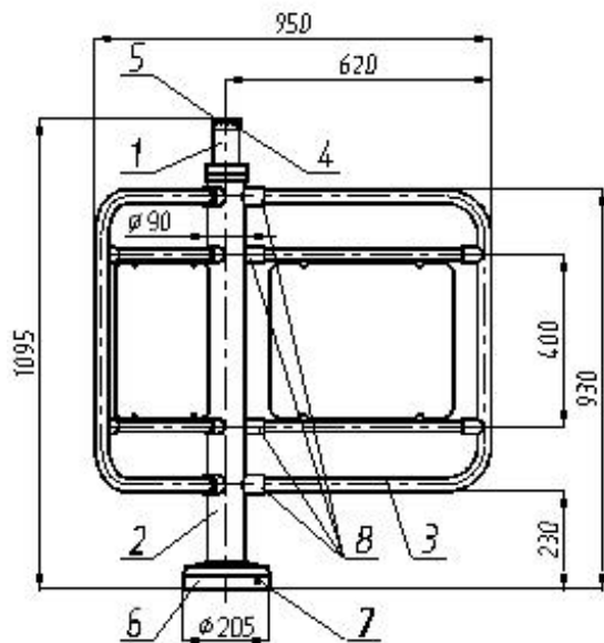
Габаритные размеры роторного турникета Р2М1/3
