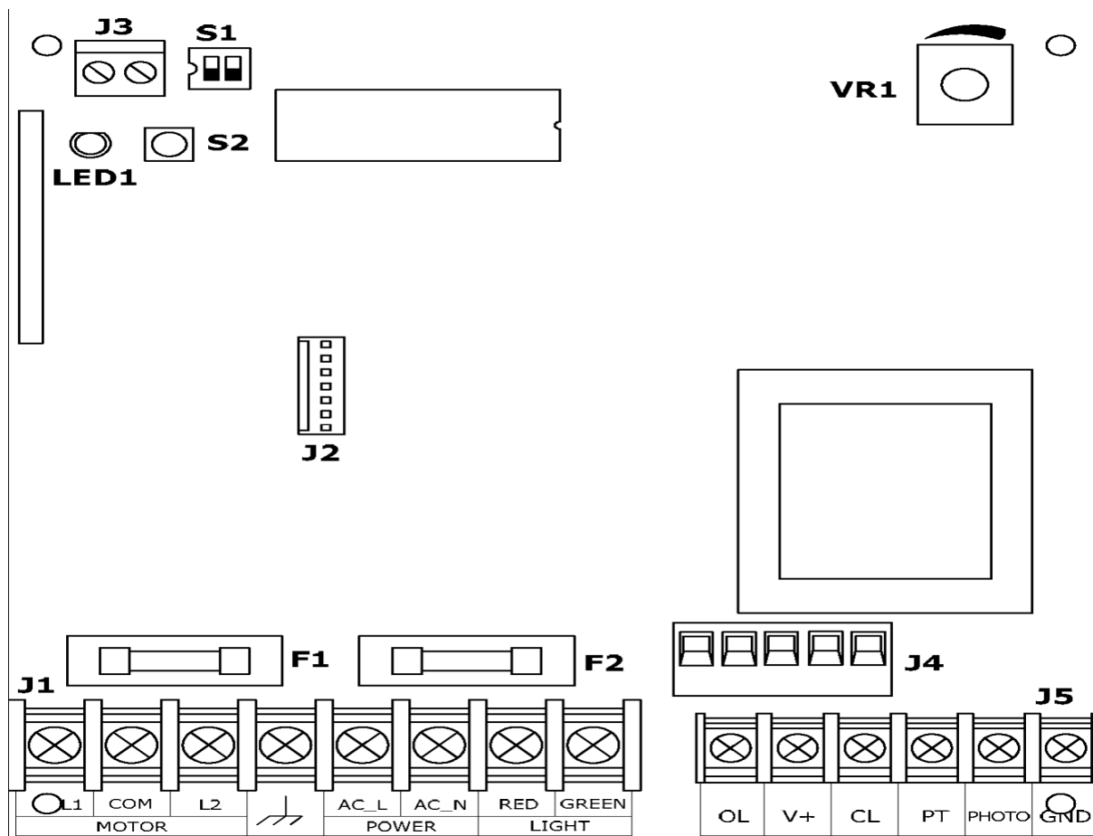
Рис. 5. Электронный модуль блока управления
