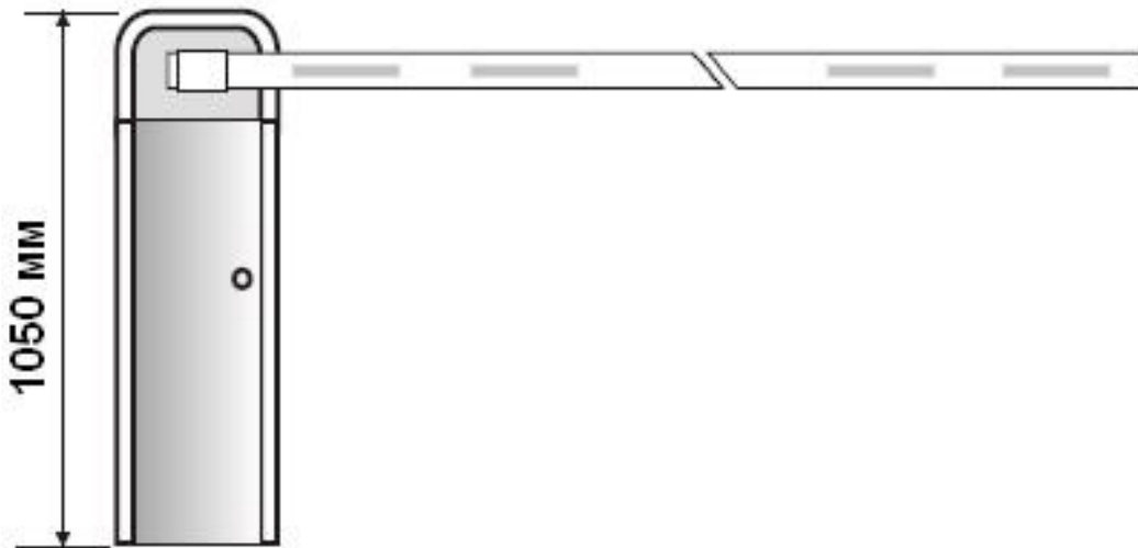
Рис. 1. Размеры илазбаума (указанны в миллиметрах)
