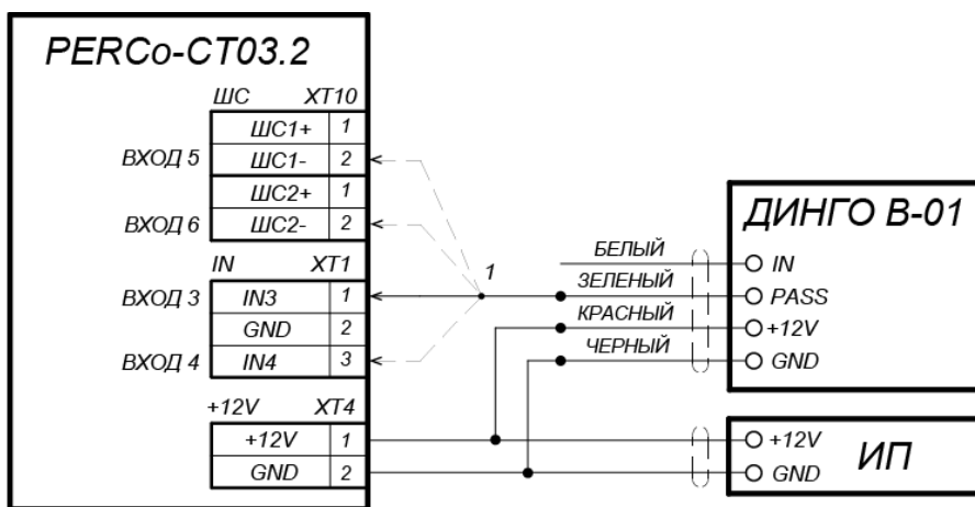
Рисунок 17. Схема подключения алкотестера «Динго В-01» (ООО СИМС-2)
