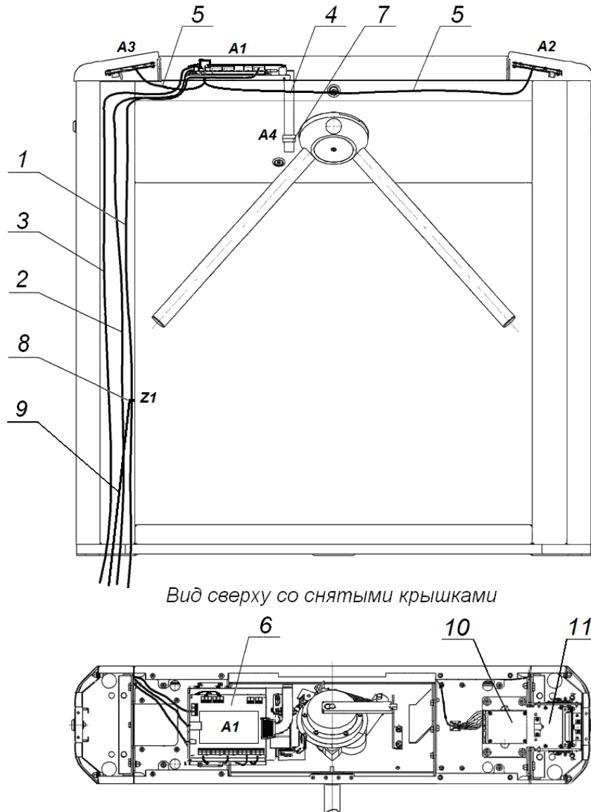
Рисунок 12. Схема прокладки кабелей в стойке ЭП
