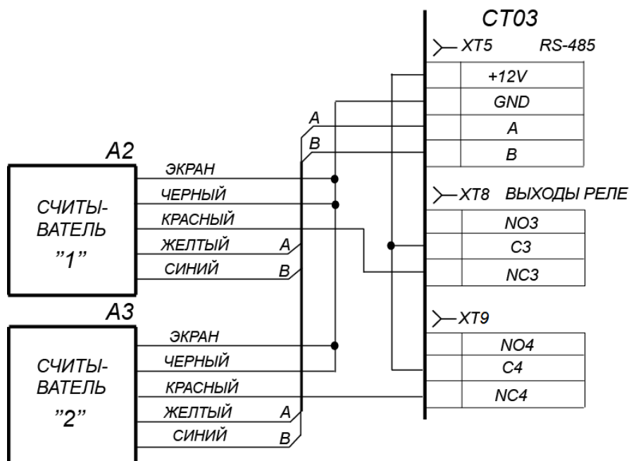
Рисунок 19. Схема подключения считывателей
