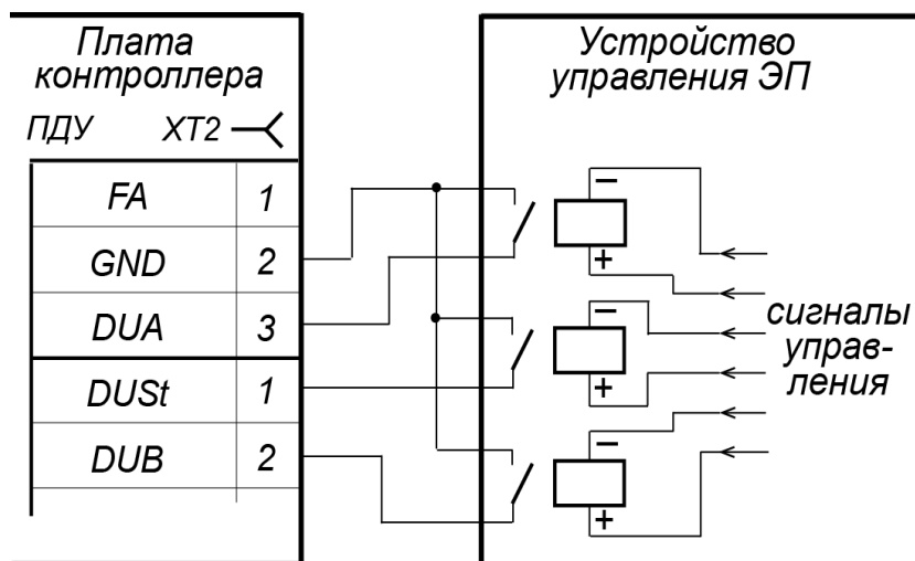
Рисунок 8. Управляющие элементы устройства управления ЭП: нормально разомкнутый контакт реле
