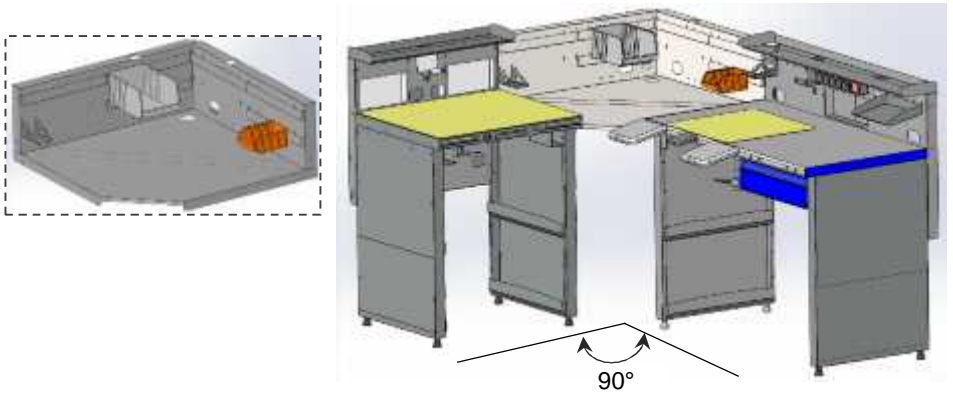
Рис.2 Пример крепления Полки к столам
