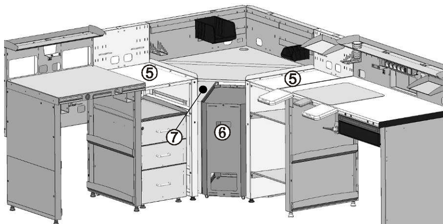
Рис.4 Пример максимального заполнения угловой зоны под Полкой – установка одного СТЕЛЛАЖ ДИРЕКТ (6) и двух СТЕЛЛАЖ КОНЕР (7)
