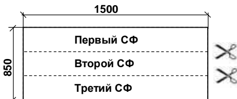
Рис.3 Пример раскроя для АМФ 1.1 / УПЗ 5.0 / УПЗ СТАЙЕР
