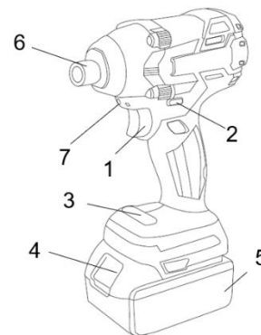
Рисунок 1.1. Устройство изделия.
