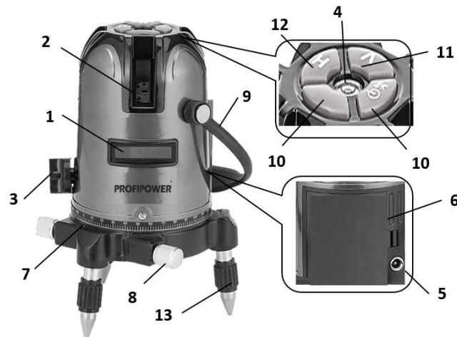
Рисунок 1.1. Устройство изделия.
