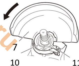
Рисунок 2.2.2. Установка защитного кожуха.
