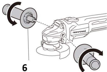
РИСУНОК 2.2.3. Установка боковой рукоятки.
