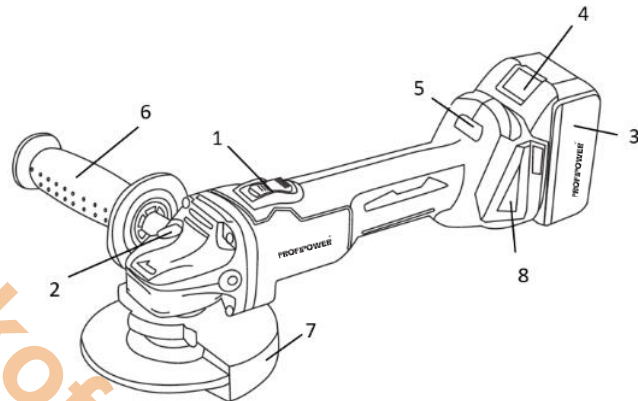
Рисунок 1.1. Устройство изделия.
