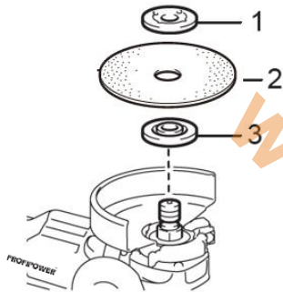
Рисунок 2.2.5. Установка оснастки.
