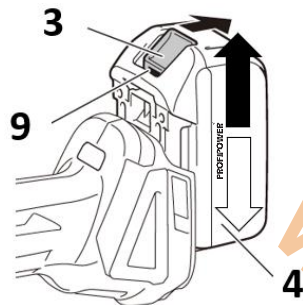
Рисунок 2.2.1. Установка и снятие аккумуляторного блока.
