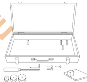
Рисунок 1.1. Устройство изделия.
