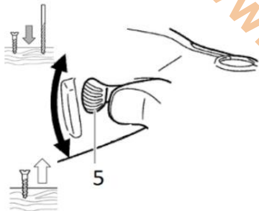
РИСУНОК 2.3.2. УСТАНОВКА НАПРАВЛЕНИЯ ВРАЩЕНИЯ.
