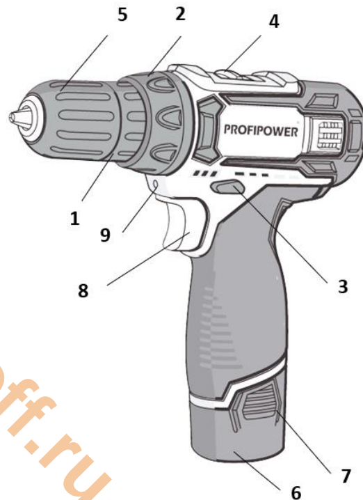
РИСУНОК 1.1. УСТРОЙСТВО ИНСТРУМЕНТА.
