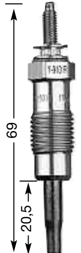
Y-910 R M 12 x 1.25 12 Hex 11,5 V
