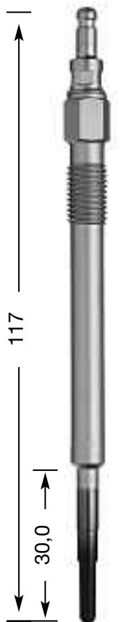
CZ 304 M 8 x 1.0 8 Hex 7 V DP 55
