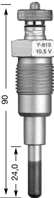
Y-810 M 18 x 1.5 20.6 Hex 10,5 V
