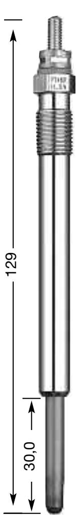
Y-746 R M 10 x 1.0 10 Hex 11,5 V
