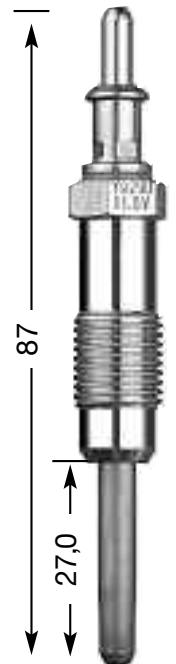
Y-929 U M 12 x 1.25 12 Hex 11,5 V DP 41
