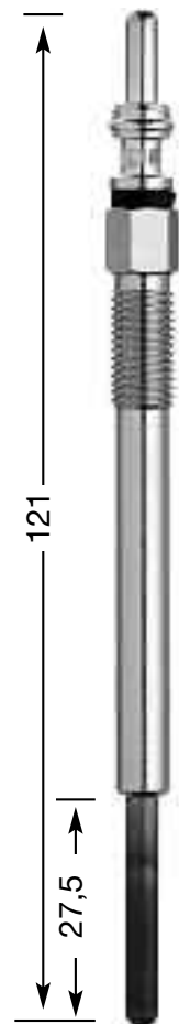
Y8003 J M 8 x 1.0 8 Hex 11 V DP 62
