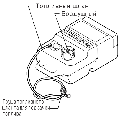
ТОПЛИВНЫЙ БАК
