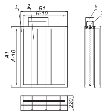
Клапан КДМ-3-СЛ электромеханическим приводом
