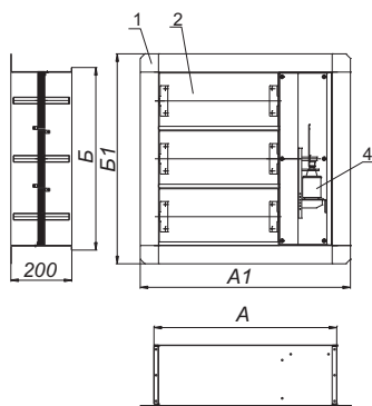
Клапан КДМ-3-СЛ электромагнитным приводом
