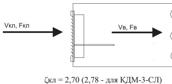
Рисунок 4. Торцевой вход в воздуховод (шахту) через клапан КДМ-3 с декоративной решеткой
