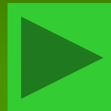
Осевая симметрия
