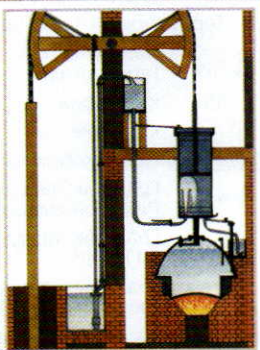
Паровой насос Ньюкомена
