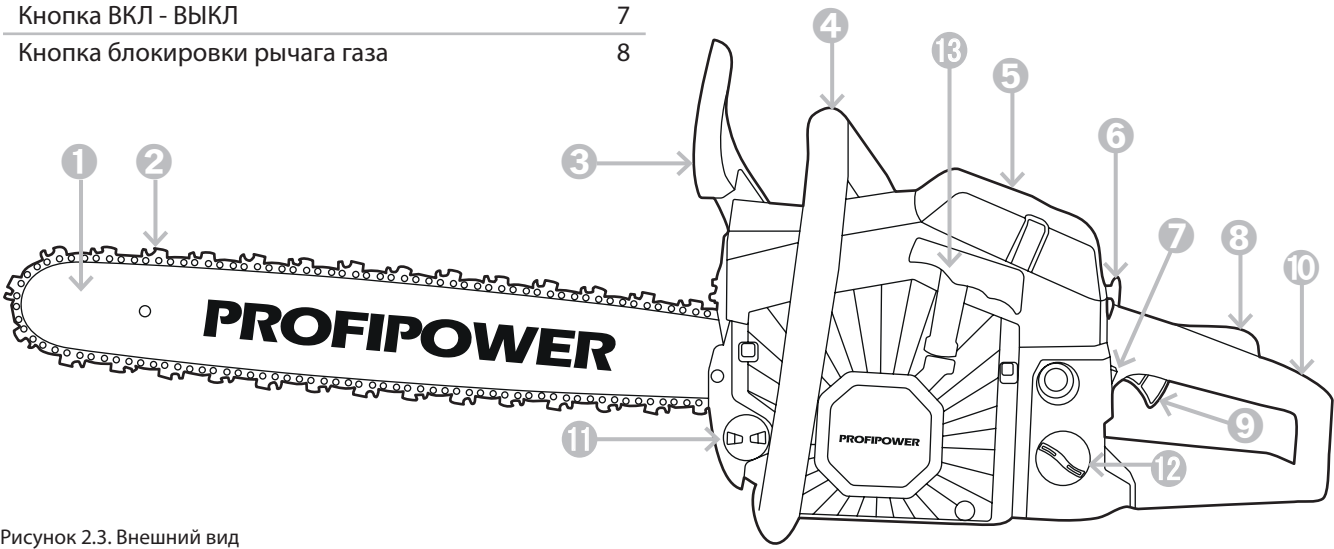
Рисунок 2.3. Внешний вид
