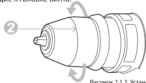
Рисунок 2.1.2. Установка оснастки
