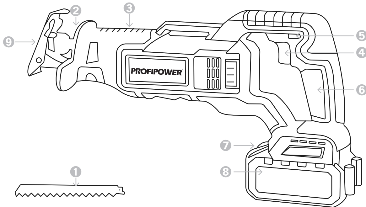
Рисунок 1.1. Устройство инструмента
