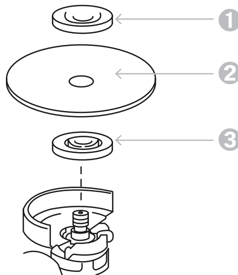
Рисунок 2.2.3. Установка оснастки
