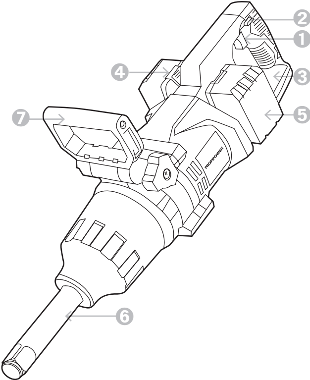
Рисунок 1.4.1. Устройство инструмента
