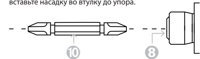
Рисунок 2.2.4. Установка насадки
