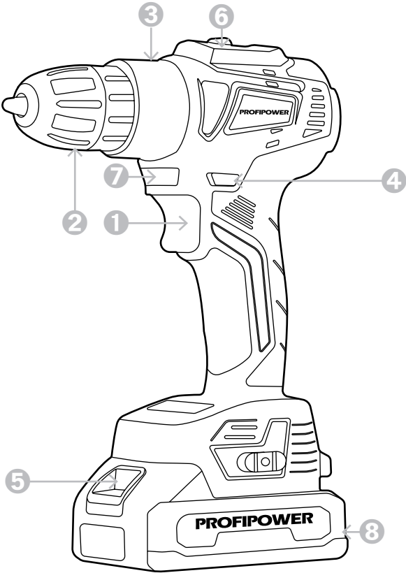
Рисунок 1.1. Устройство инструмента
