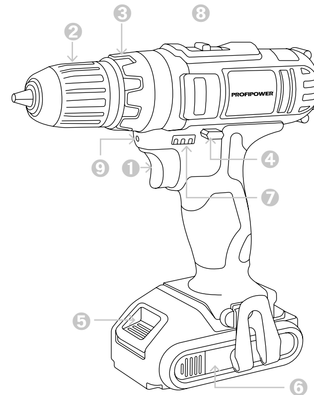
Рисунок 1.1. Устройство инструмента
