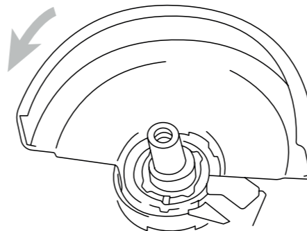
Рисунок 2.2.5. Установка защитного кожуха
