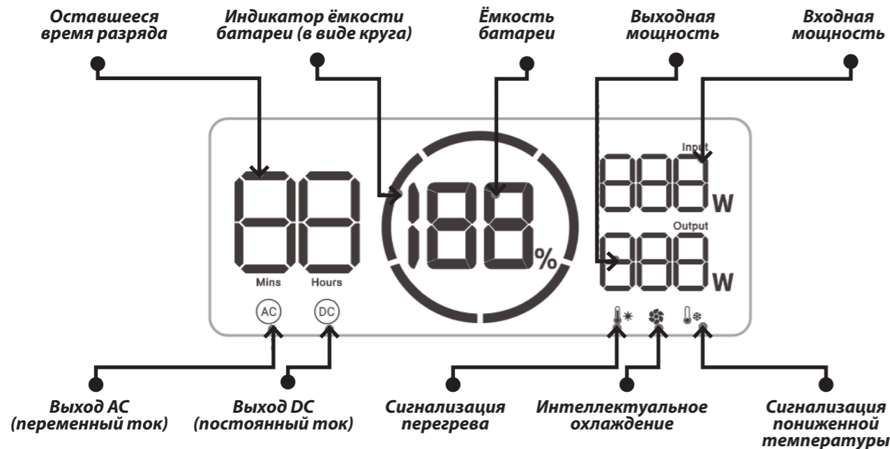
Рисунок 1.5.1. ЖК-экран
