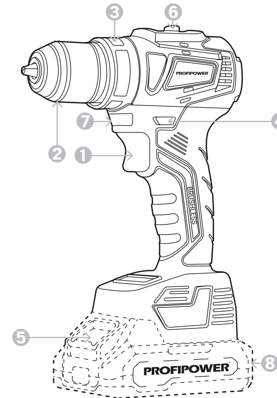
Рисунок 1.1. Устройство инструмента
