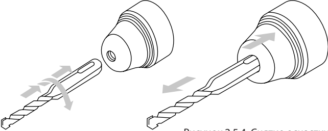
Рисунок 2.5.4. Снятие оснастки
