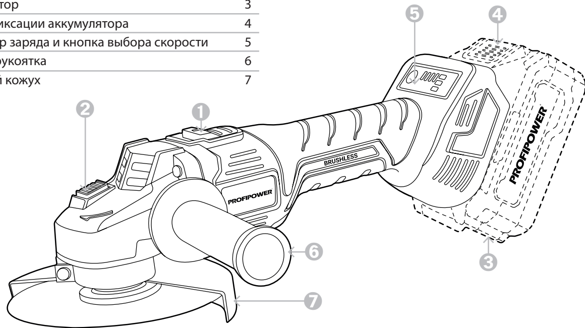
Рисунок 1.4.2. Устройство инструмента
