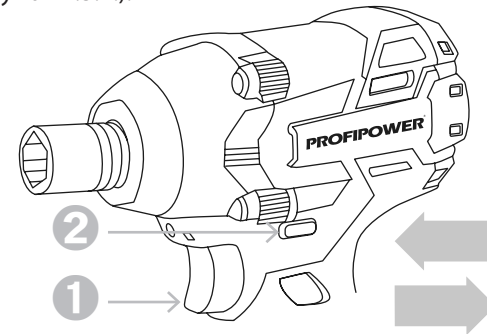
Рисунок 2.3.7. Установка направления вращения
