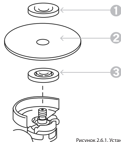
Рисунок 2.6.1. Установка оснастки
