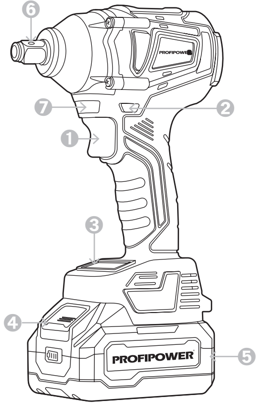
Рисунок 1.4.1. Устройство инструмента
