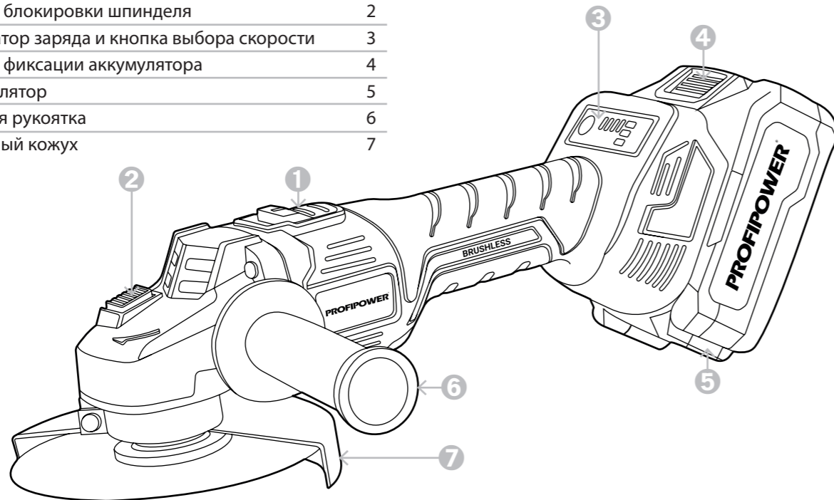
Рисунок 1.6.1. Внешний вид УШМ
