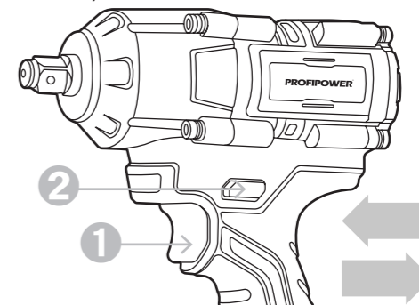
Рисунок 2.3.7. Установка направления вращения
