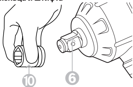
Рисунок 2.3.2. Установка головки
