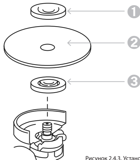
Рисунок 2.4.3. Установка оснастки
