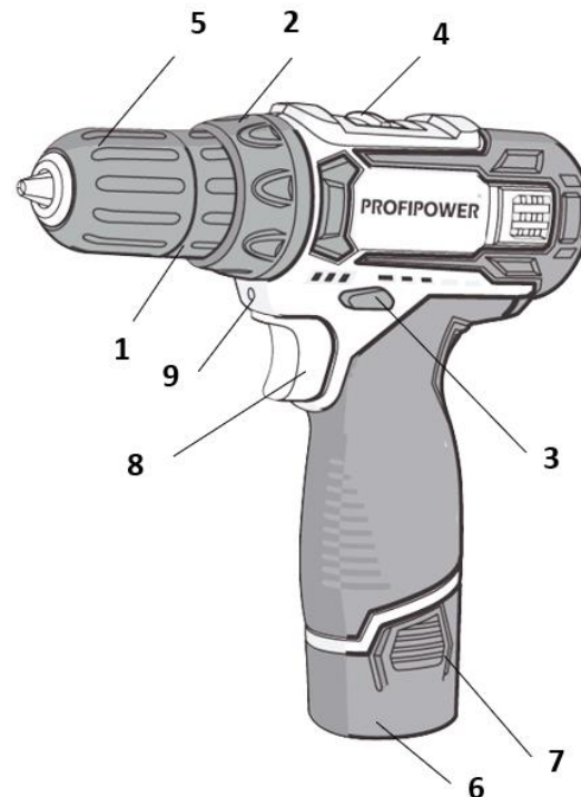
РИСУНОК 1.1. УСТРОЙСТВО ИНСТРУМЕНТА.
