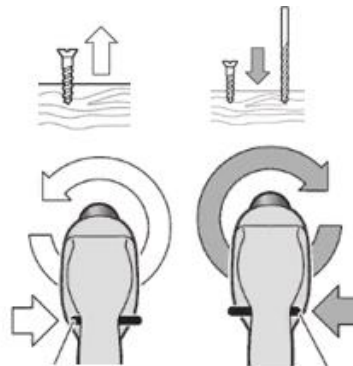
РИСУНОК 2.3.1. УСТАНОВКА НАПРАВЛЕНИЯ ВРАЩЕНИЯ.
