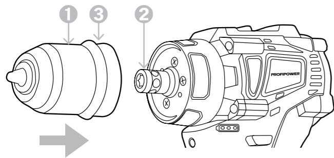
Рисунок 2.2.3. Установка патрона
