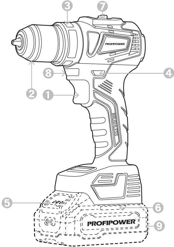
Рисунок 1.4.4. Устройство инструмента
