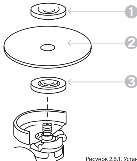
Рисунок 2.6.1. Установка оснастки
