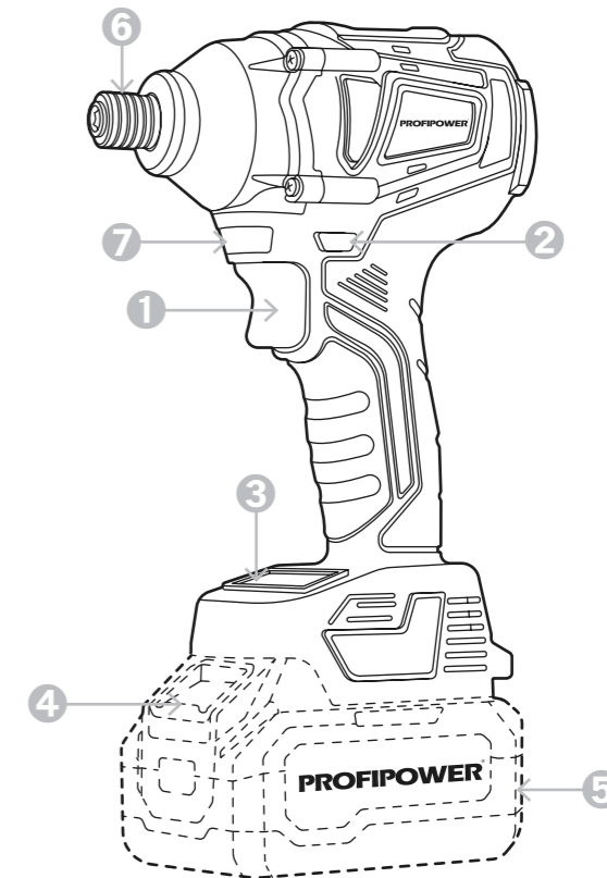
Рисунок 1.1. Устройство инструмента
