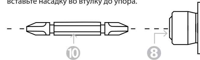
Рисунок 2.2.4. Установка насадки
