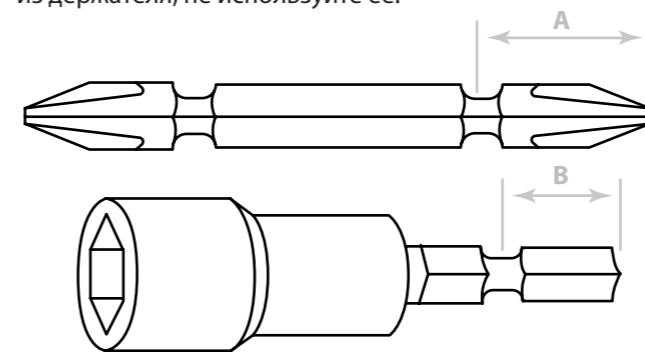
Рисунок 2.2.3. Типы рекомендуемых насадок
