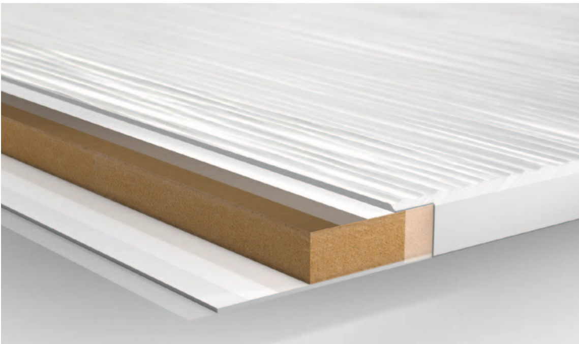
Плита Wave в разрезе
