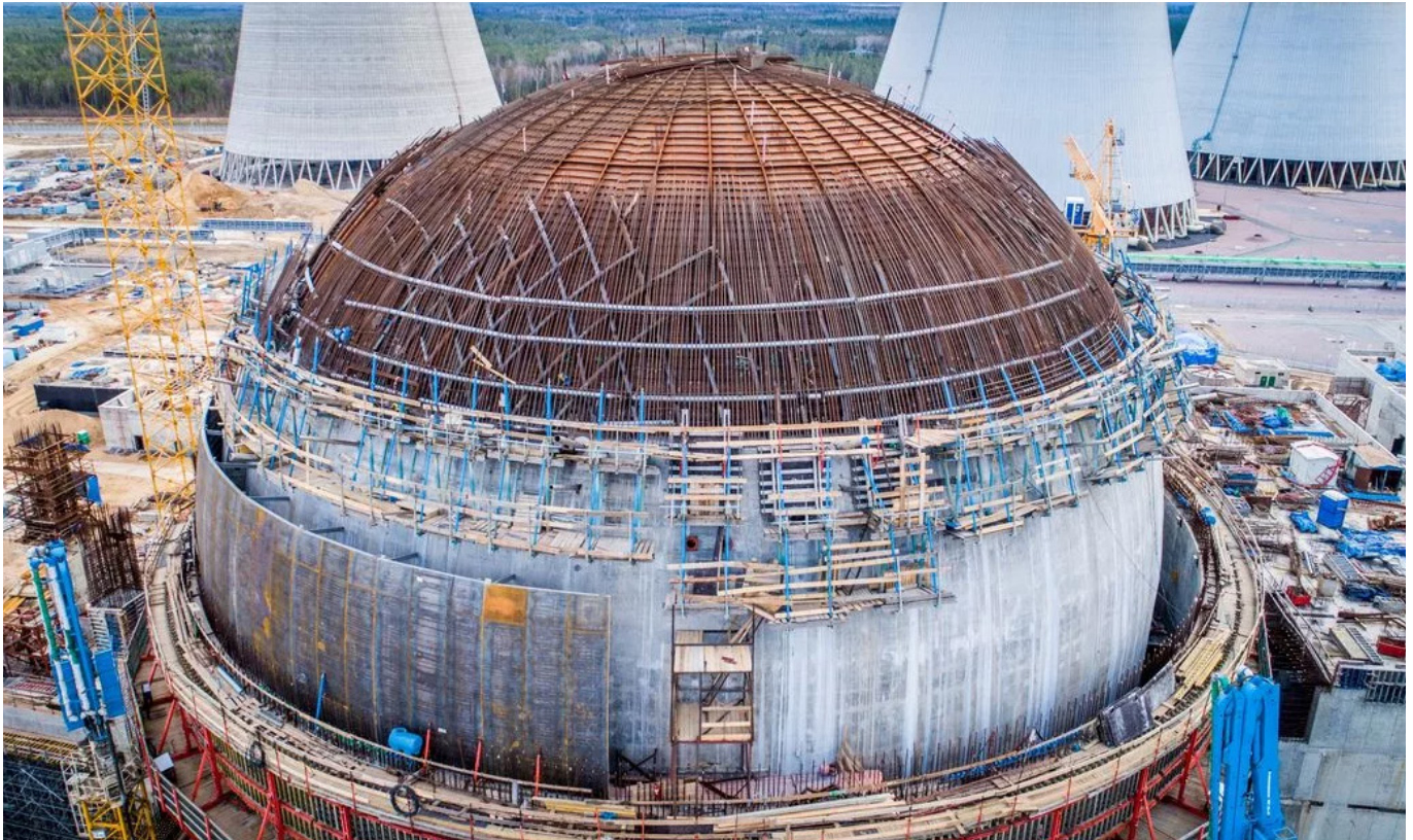
Рисунок 5.1.2 — Здание реактора
