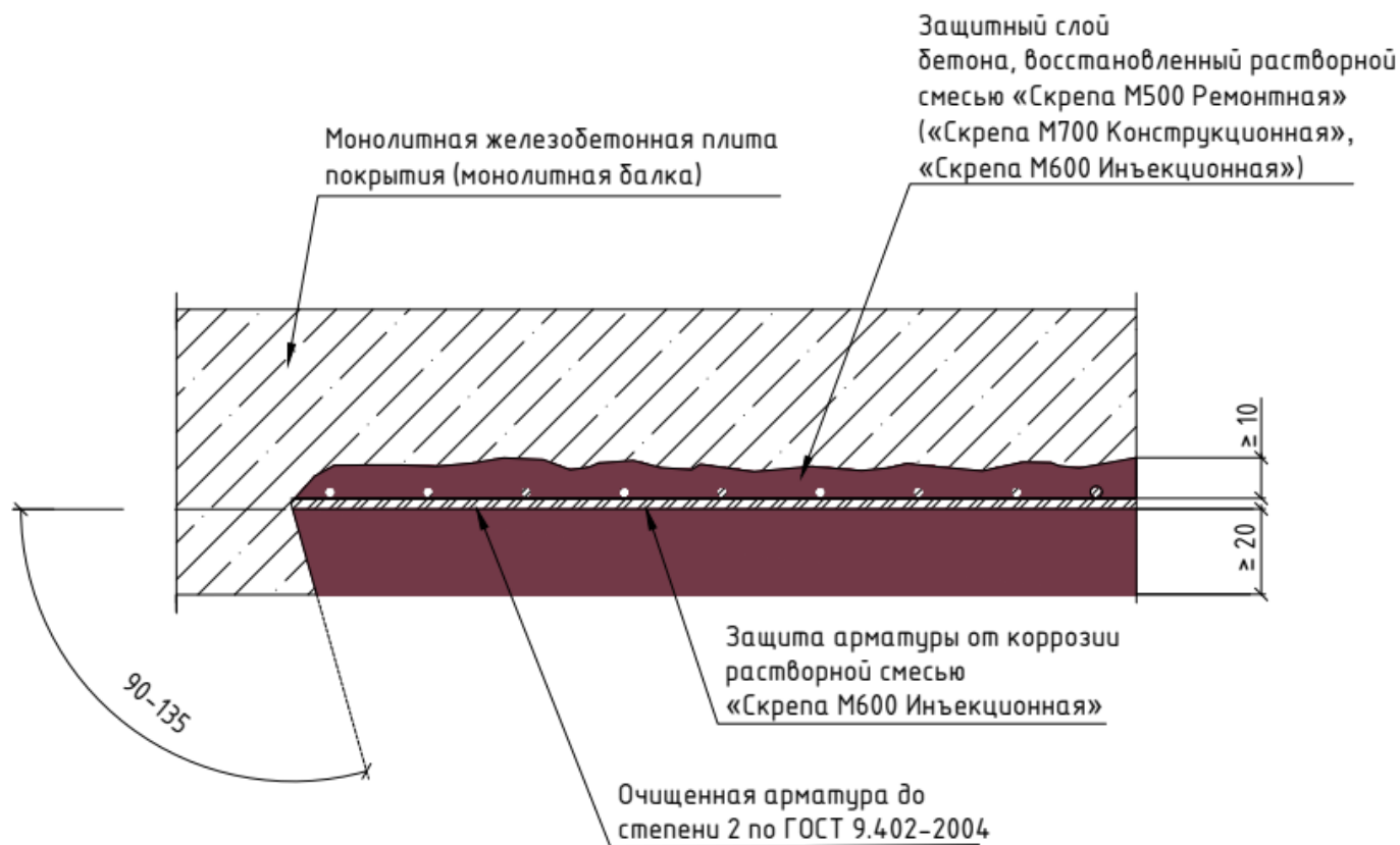
Рисунок 8.3.3.2 — Схема восстановления потолочных поверхностей
