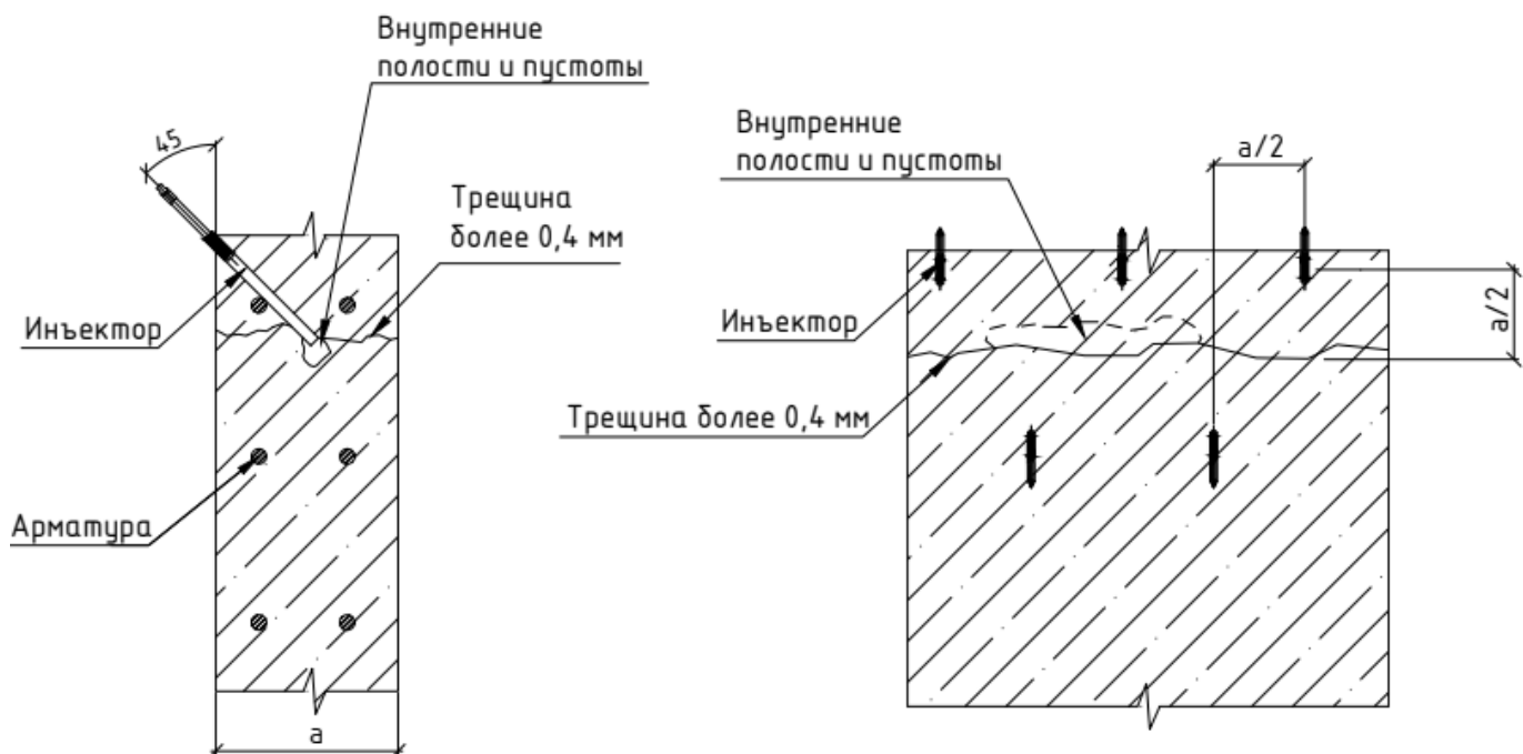
Рисунок 8.3.4.1 — Схема установки инъекторов
