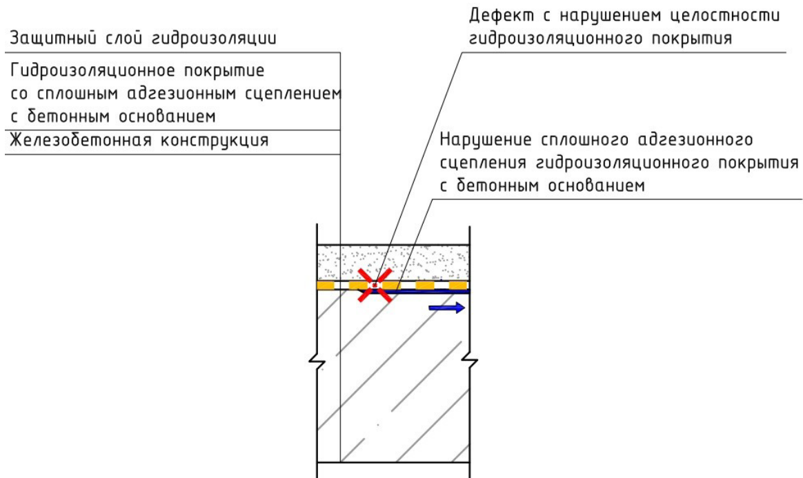
Рисунок 4.2.3 — Дефекты гидроизоляционного покрытия с миграцией воды по изолируемой бетонной поверхности
