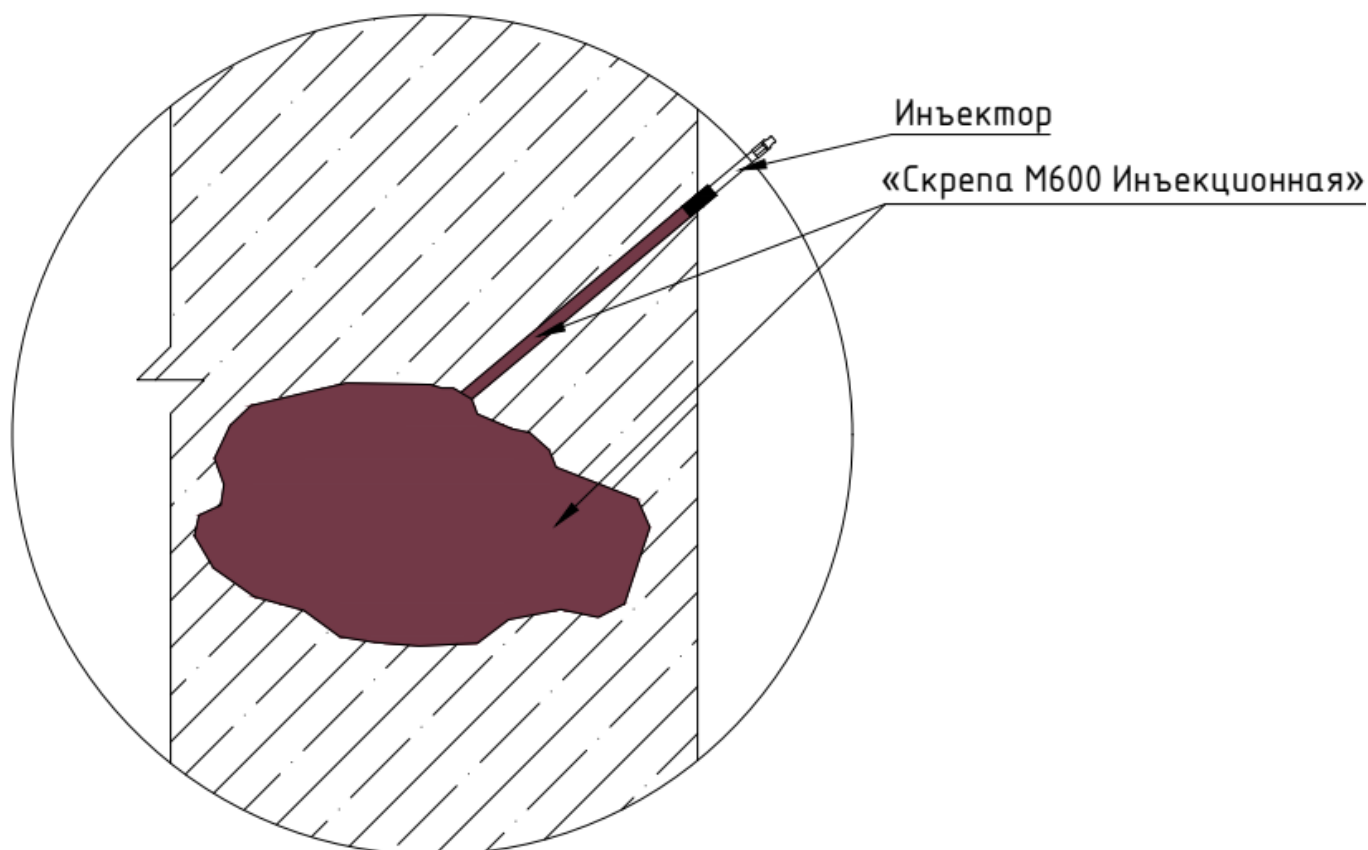
Рисунок 8.3.4.3 — Схема заполнения пустот и полостей
