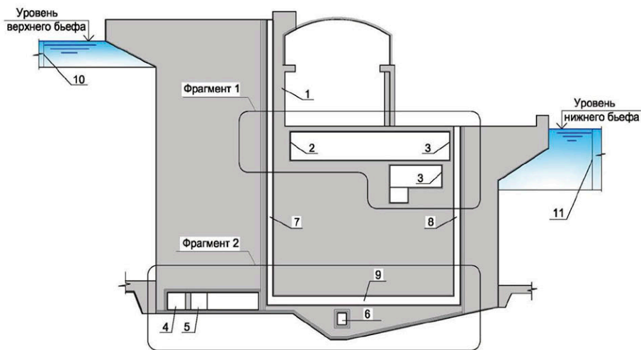
Рисунок 6.1.1 - Русловое здание ГЭС:
