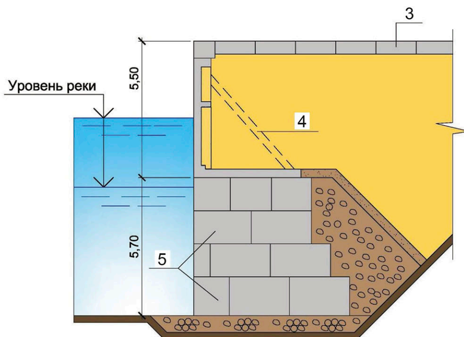
Рисунок 6.5.2 - Конструкция причального сооружения из массивной кладки с надстройкой: 3 - бетонное покрытие; 4 - уголковая надстройка из сборного железобетона; 5 - бетонные массивы.
