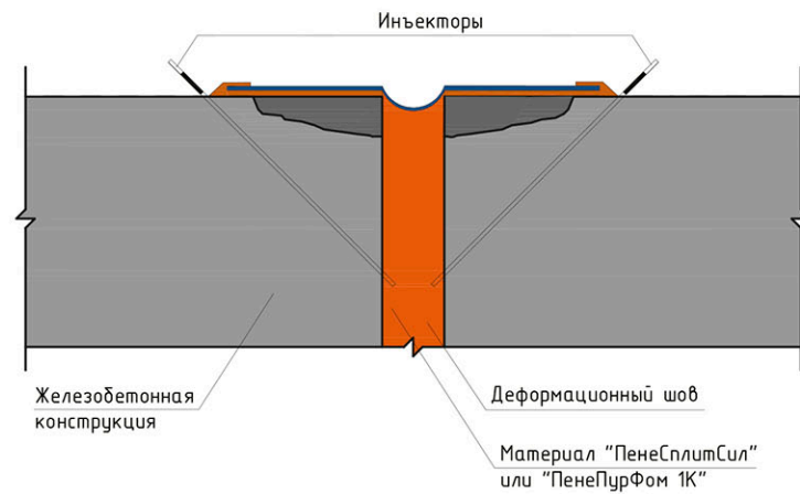
Рисунок 7.3.15 - Заполнение полости шва ињекционными смолами.
