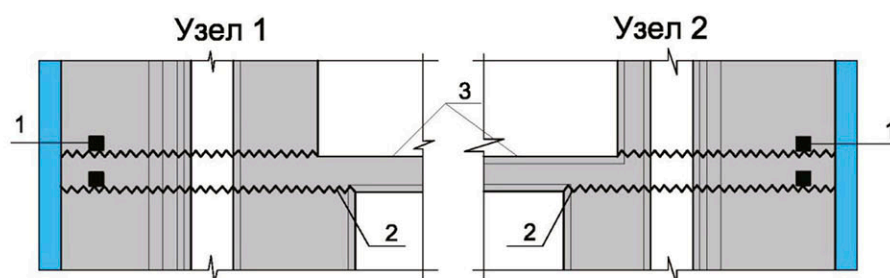
Рисунок 7.1.9 – Типовые узлы гидроизоляции в машинном зале технологических помещениях (узлы 1 и 2 на рис. 7.1.8):
