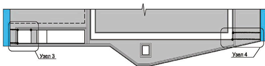
Рисунок 7.2.7 - Гидроизоляция швов бетонирования и швов сопряжения стен и перекрытий в потернях, смотровых шахтах и соединительных коридорах здания ГЭС (фрагмент 2 на рис. 6.1.1).
