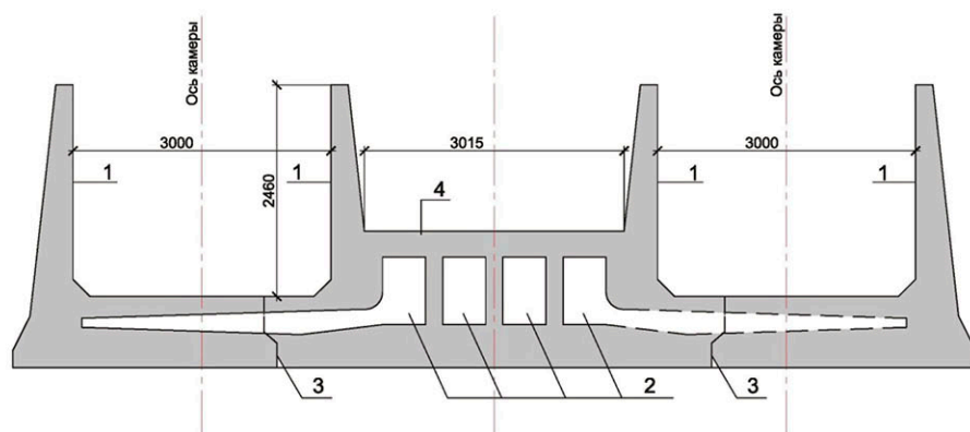
Рисунок 6.3 - Двухниточный судоходный шлюз: а - общий вид: слева - эксплуатируемая камера; справа - осушенная камера; б - поперечный разрез по камерам; 1 - стены судоходных камер; 2 - водопропускные галереи; 3 - деформационные швы; 4 - перекрытие водопроводных галерей.
