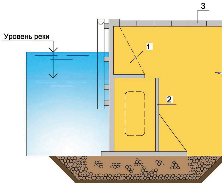
Рисунок 6.5.1 - Конструкция причального сооружения из железобетонных массивов-гигантов: 1 - контрфорсная надстройка; 2 - массив гигант; 3 - бетонное покрытие.
