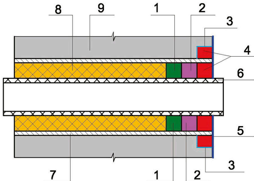
Рисунок 7.2.52а - Гидроизоляция места ввода коммуникаций: 1 - гидропломба «Пенеплаг» («Ватерплаг»); 2 - гидроизоляционный жгут «Пенебар»; 3 - грунтослойный слой «Пенетрон»; 4 - «Пенекрит»; 5 - «Пенетрон» (2 слоя); 6 - металлическая труба; 7 - металлическая гильза; 8 - сальниковая набивка; 9 - монолитный бетон конструкции.
