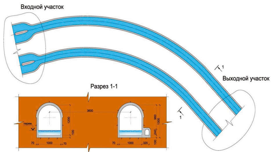
Рисунок 6.7.1 - Водосбросные туннели: а – выходной участок туннеля; б – схема трассы туннелей и поперечный разрез по туннелям.
