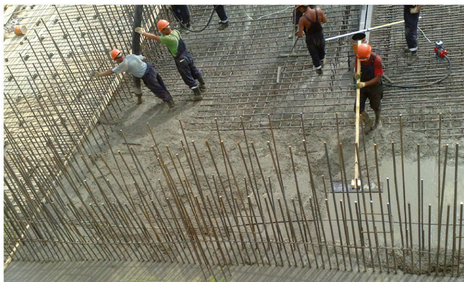
Рисунок 7.1.3 - Укладка бетонной смеси.
