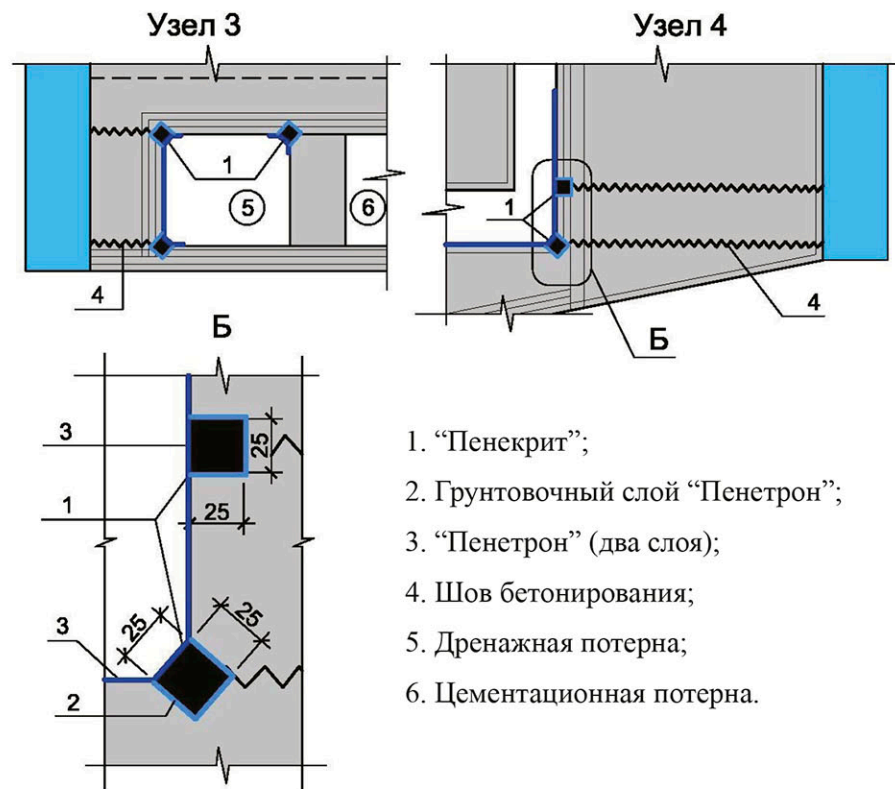
Рисунок 7.2.8 - Типовые узлы гидроизоляции в потернях, смотровых шахтах и соединительных коридорах (узлы 3 и 4 на рис. 7.2.7).
