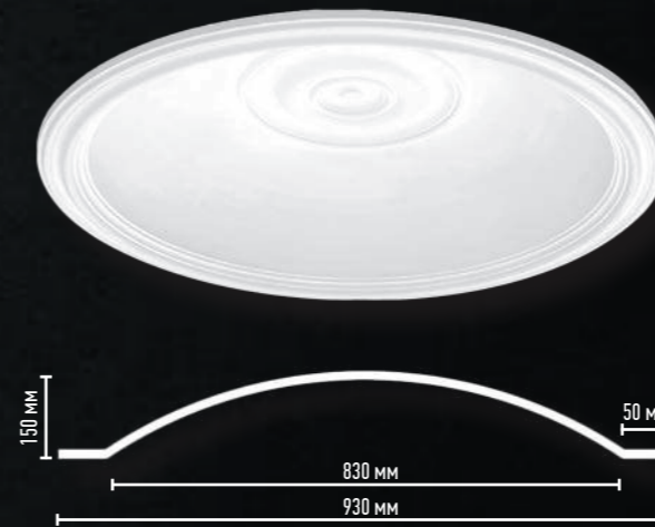
DR 63 (150 x Ø930 x 130 мм)
