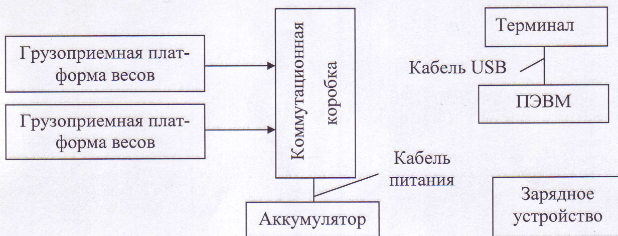
Рисунок 3б – Схема подключения весов при беспроводном соединении
