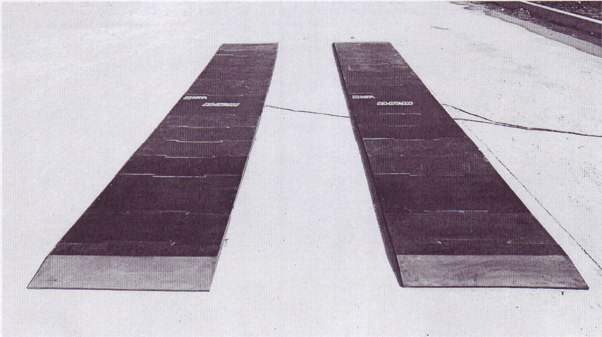
Рисунок 1 – Пример установки грузоприёмных платформ с пассивными площадками и въездными пандусами.
