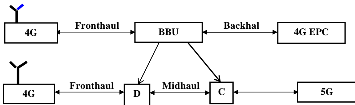
Рисунок 2. Архитектуры 5G C-RAN и 4G C-RAN высокого уровня
