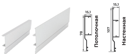
9 Накладка декоративная
