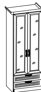
Шкаф 2-х дверный с зеркалом и ящиками 800x560x2113
