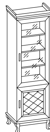
Шкаф 1 дверный остеклённый 706x465x2105
