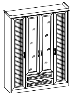
Шкаф 4-х дверный с зеркалом и ящиками 1600x560x2113
