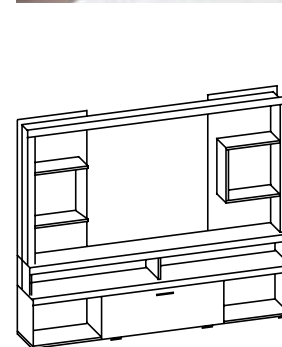
Шкаф (комбинированный) 2180x366x1773
