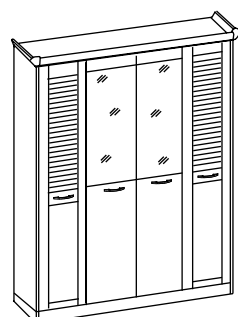
Шкаф 4-дв. 1824x582x2155
