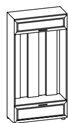
Шкаф „800” с вешалкой 800x440x2172
