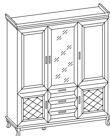
Шкаф 3-х дверный с 3-мя ящиками 1866x618x2204
