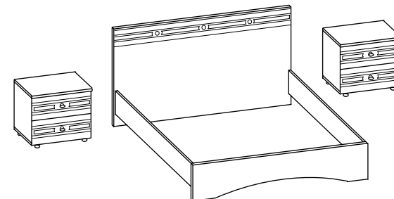
Тумба прикроватная 510x350x460
