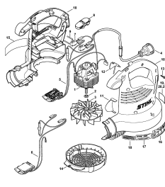
BGE 71 USA, CDN: Электродвигатель - Корпус вентилятора
