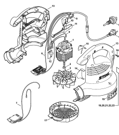
BGE 81: Электродвигатель - Корпус вентилятора
