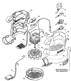
BGE 71: Электродвигатель - Корпус вентилятора
