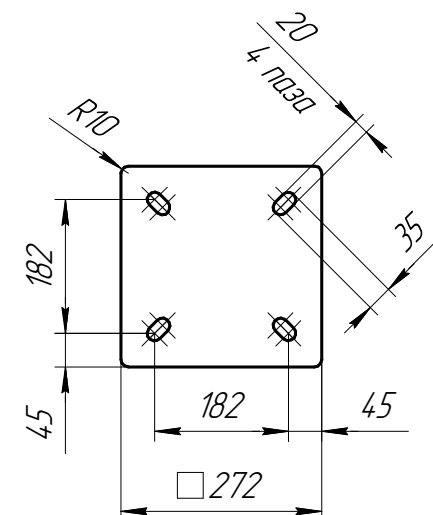
Поз.6 Опорный фланец
