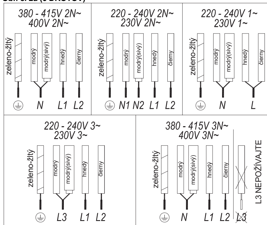
Obr. č. 2a (5 DRÔTOV)
