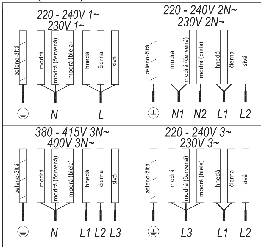
Obr. č. 2b (7 DRÔTOV)
