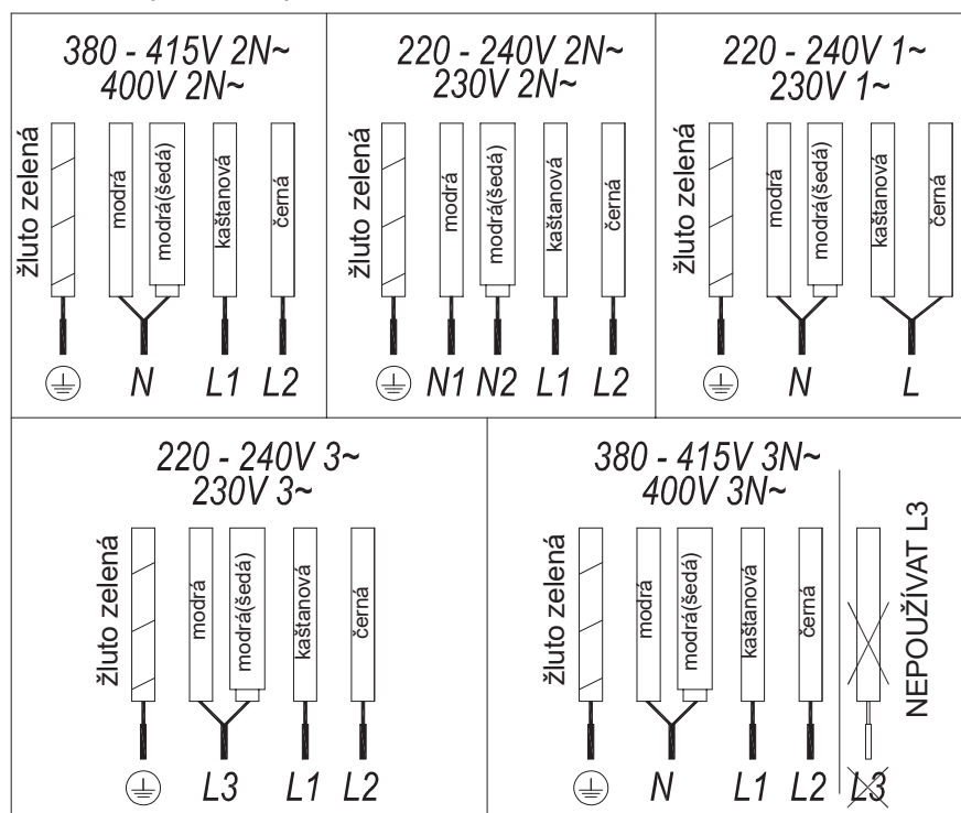
Obr. č. 2a (5 VODIČŮ)
