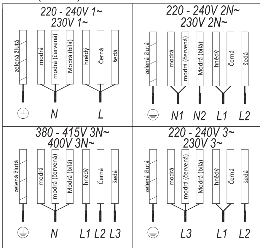
Obr. č. 2b (7 VODIČŮ)
