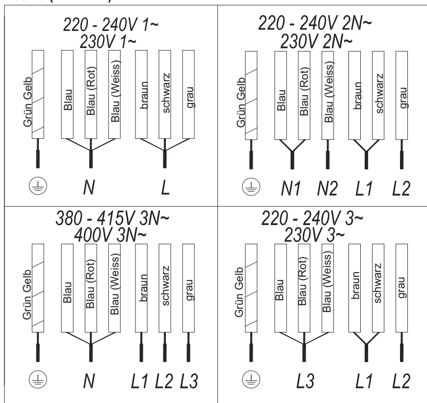
Abb.2b (7 KABEL)
