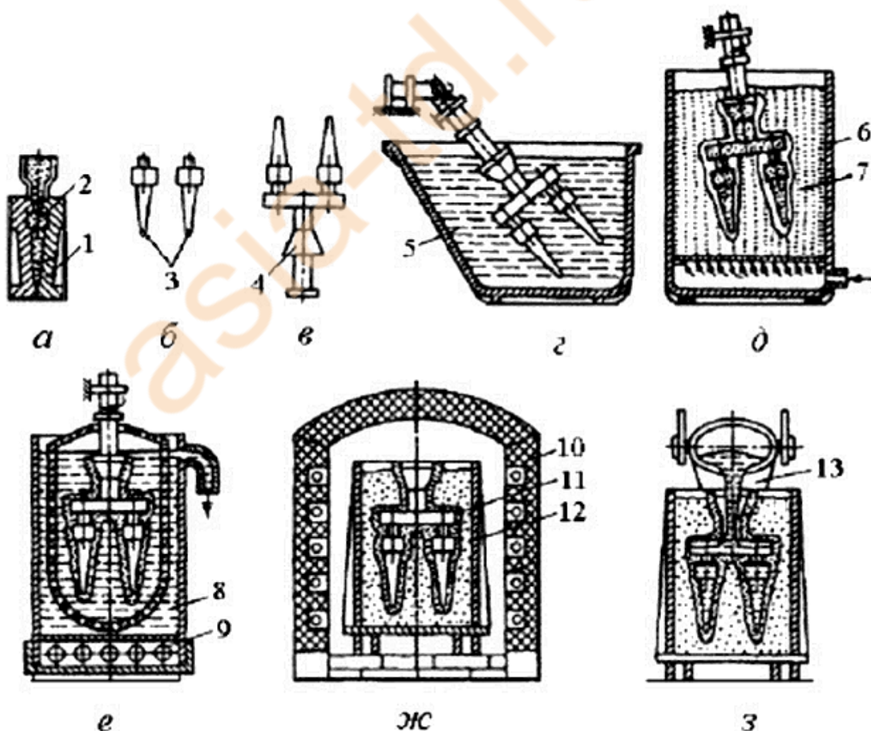
Рисунок 2.5 – Последовательность операций процесса литья по выплавляемым моделям:
