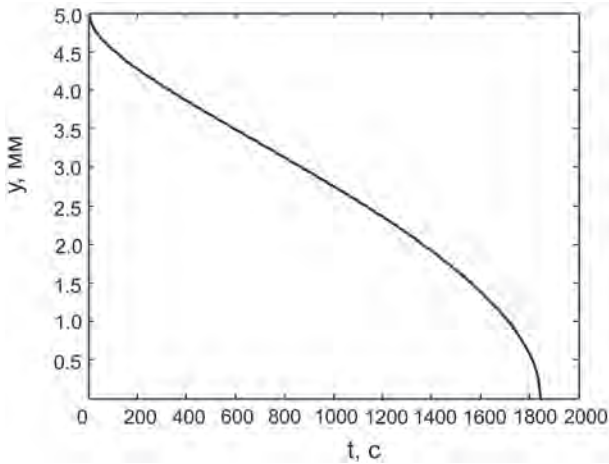
Рис. 5. Кинетика растворения сферической частицы хрома с исходным радиусом r_0 = 5 мм в медном расплаве при 1500\text{ }^\circ\text{C}
