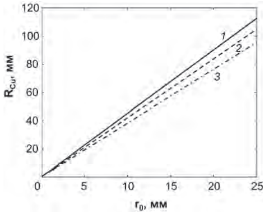
Рис. 2. Радиус эквивалентной сферы медного расплава вокруг твердых частиц хрома с учетом угара u : 1 – u = 0,1 ; 2 – 0,3 ; 3 – 0,5
