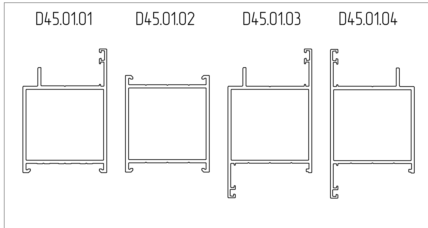
04_Штапики
