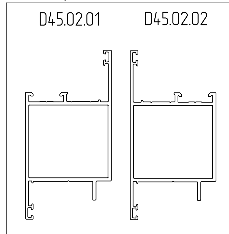
02_Створки
