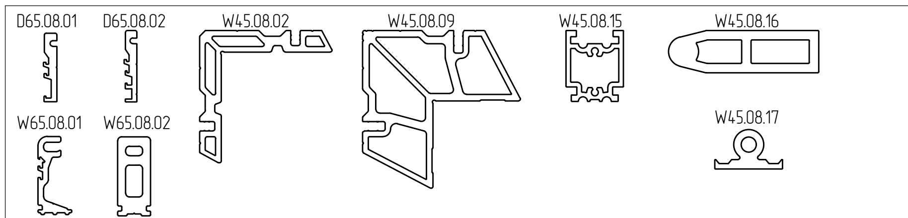
10_Уплотнители
