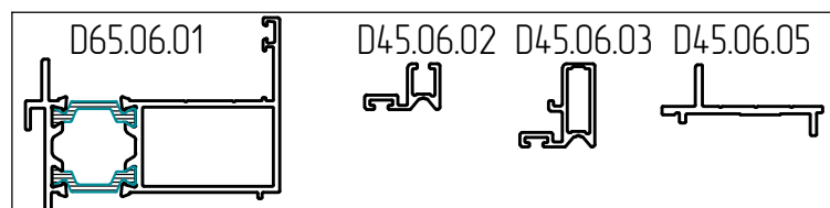
06_Адаптеры
