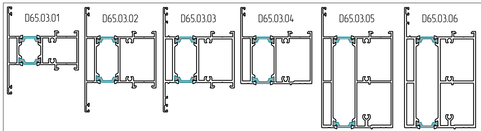
04_Штанги
