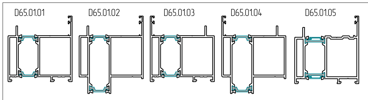
01_Рамы
