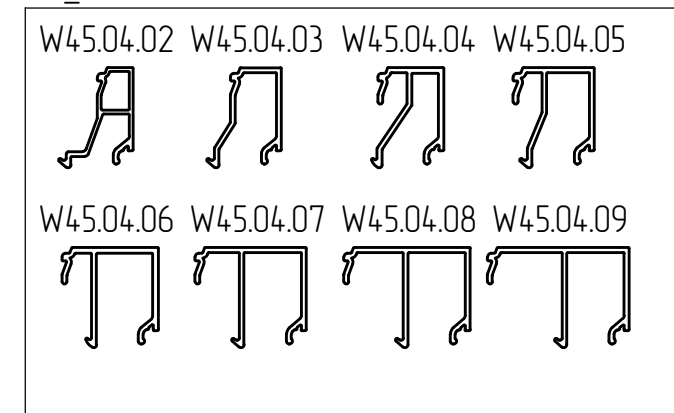
04_Штанги
